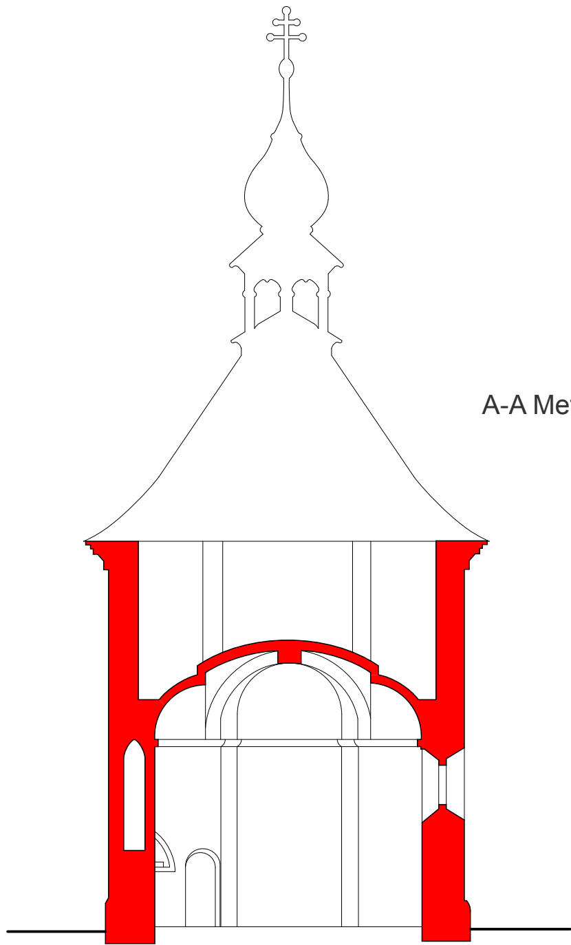
A templom keresztmetszete és alaprajza
