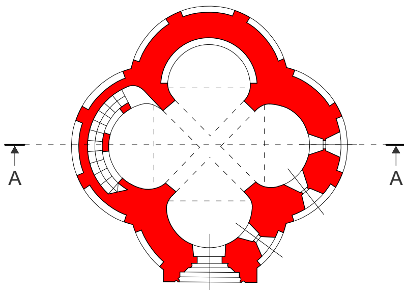
A templom keresztmetszete és alaprajza
